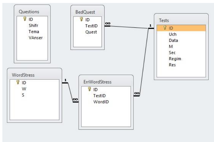
Рисунок 4.1 – Схема бази даних
